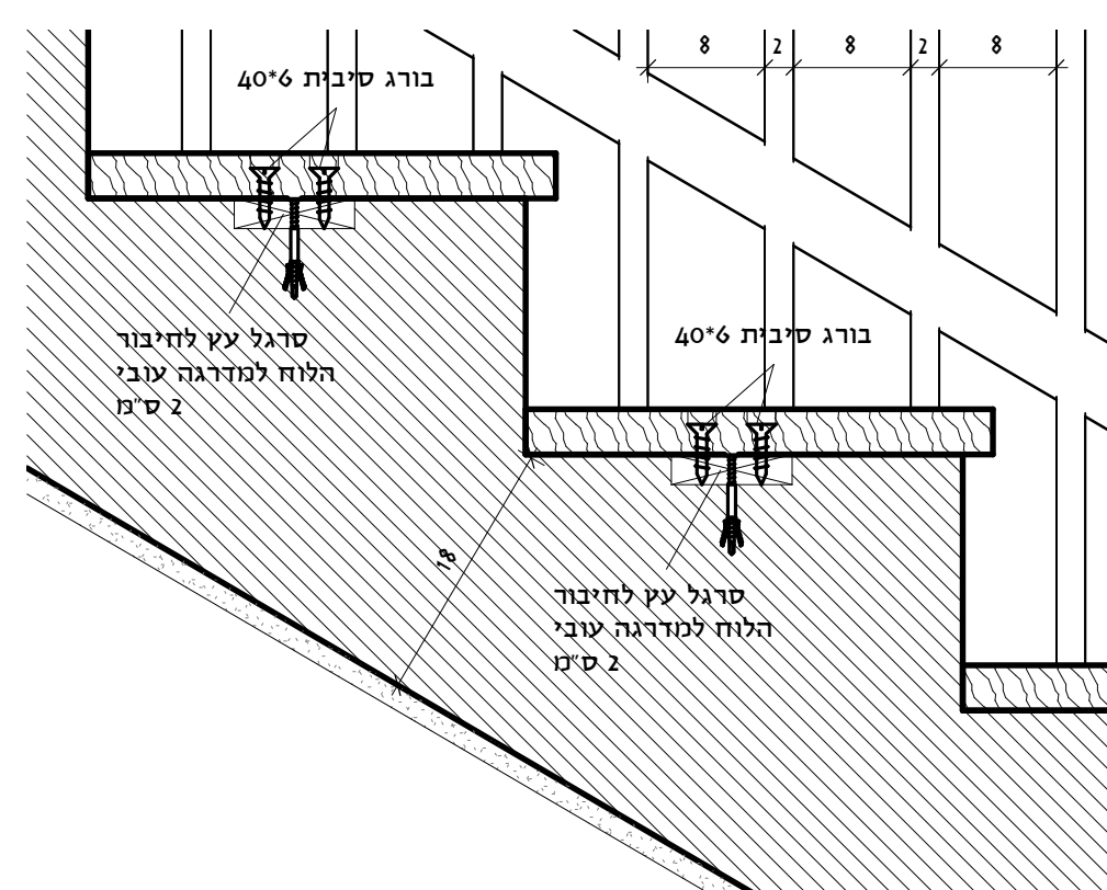
פרט מדרגה 1:5 (3)
