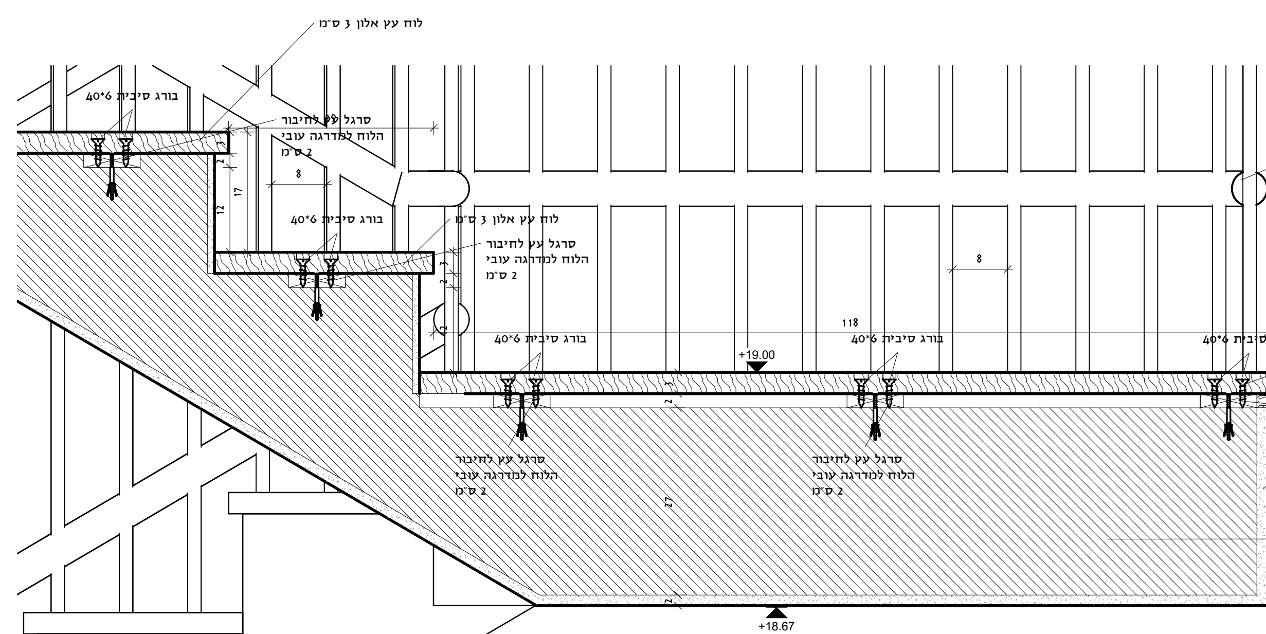
פרט חיבור מדרגות לפודסט 1:5 (5)
