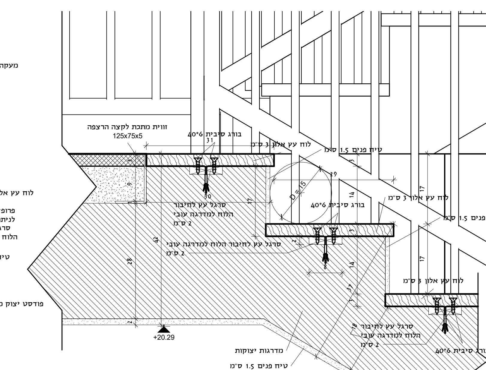
פרט חיבור מדרגה לרצפה 1:5
