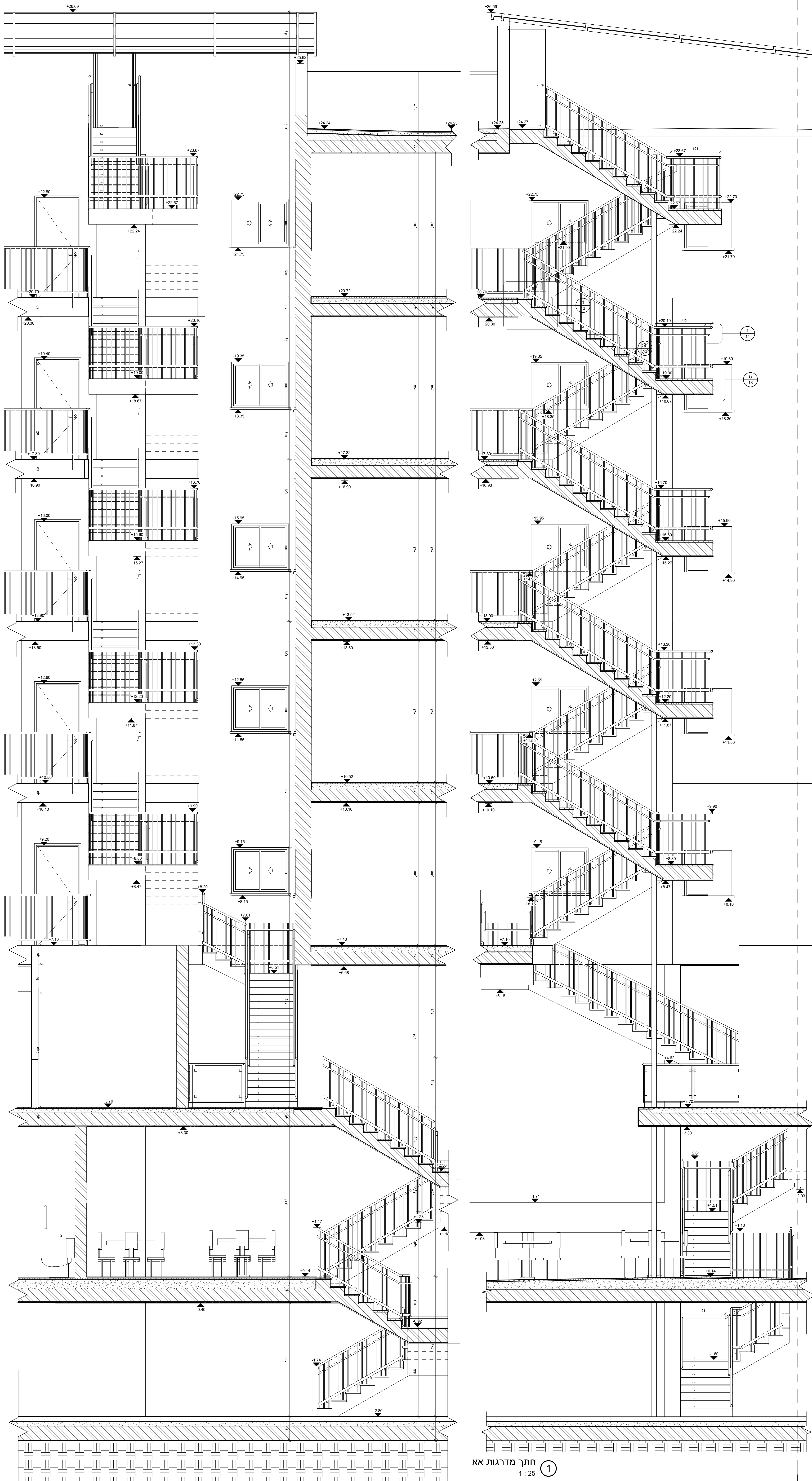
חֵתֶךְ מִדְּרָגוֹת בֵּב (2) 1 : 25
